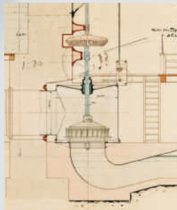
Projektplan für eine Francis- turbine der Firma Rieter & Cie. Winterthur für die Spinnerei Blumer, 1904.
